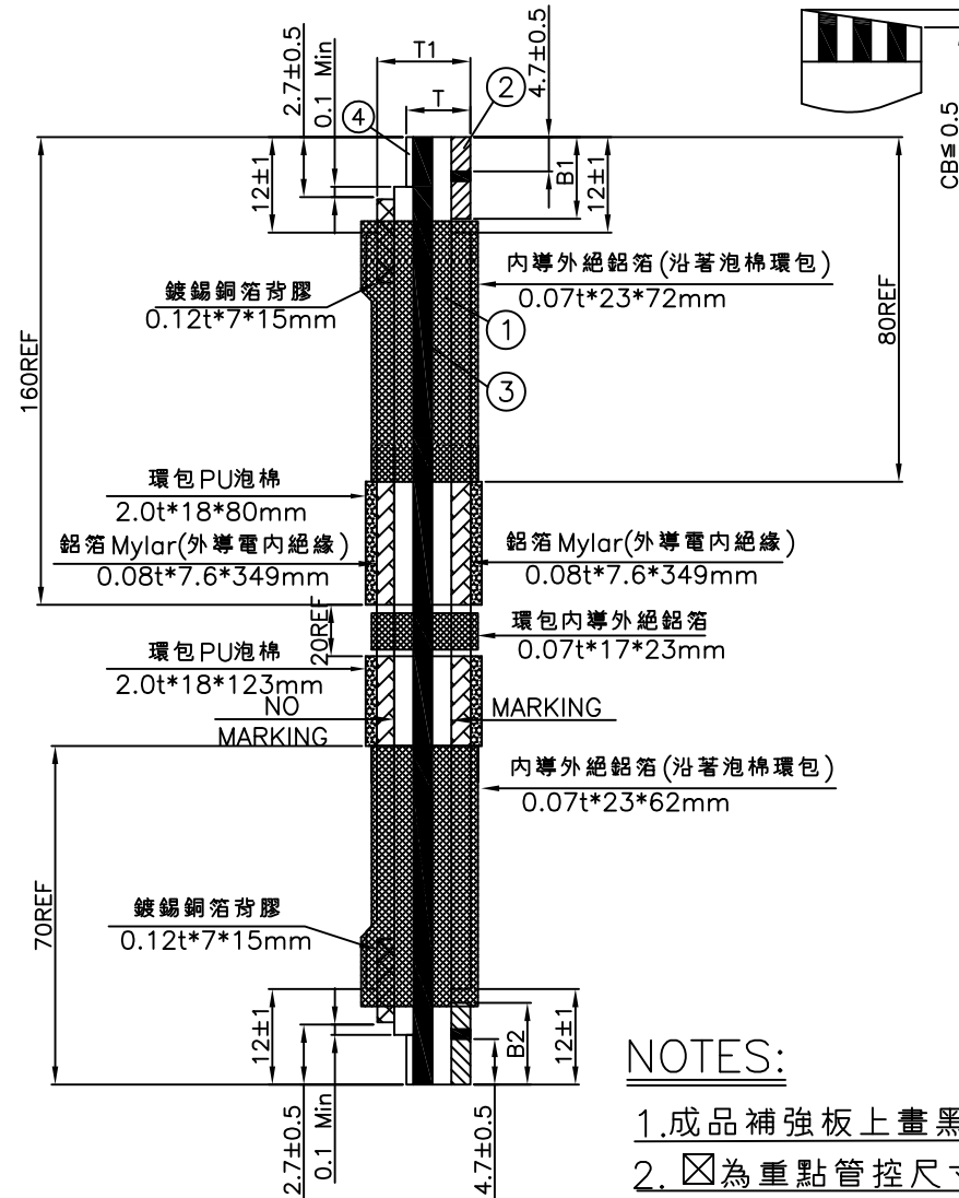
SECTION A-A
